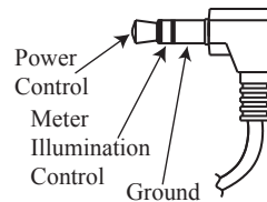
Figure 12– Power Control (trigger) mini plug
