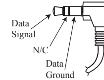
Figure 13– Data Out mini plug
